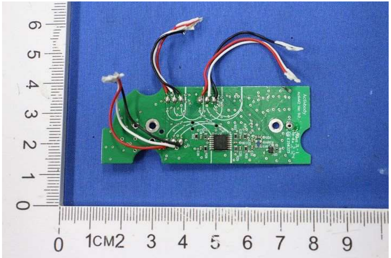
PCBA (1)
