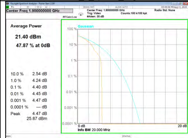
Band2_1_Q16_High
