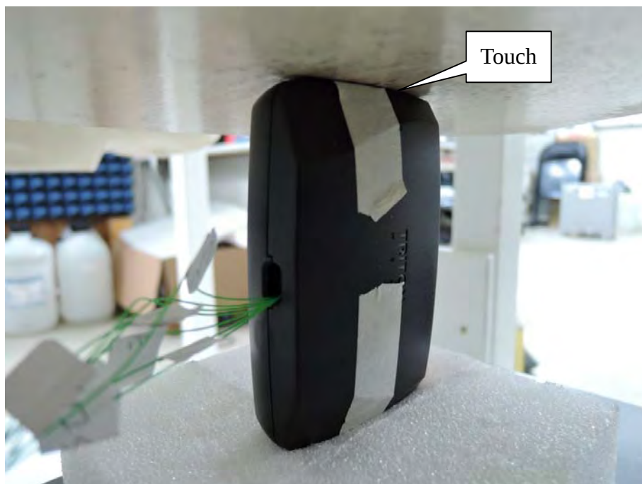
EUT Left-Side (BLE)
