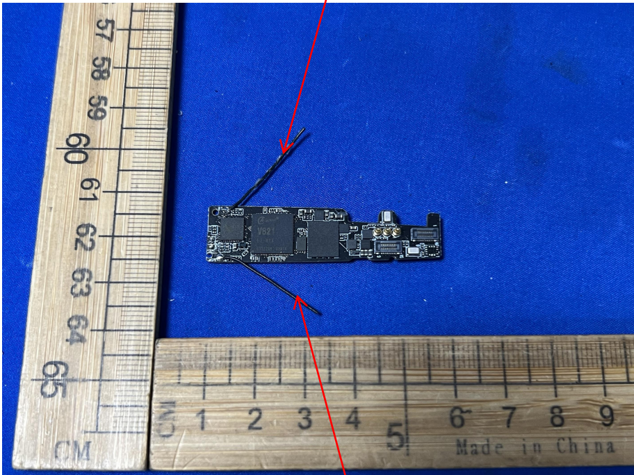
WLAN ANT
