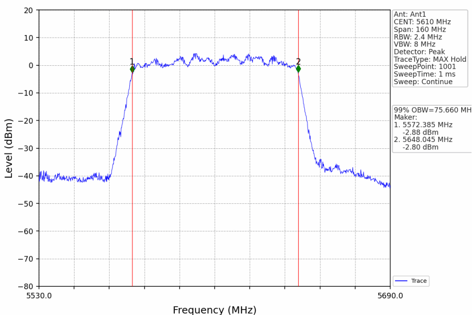
802.11ac(VHT80)_HCH_5610MHz_Ant1_NTNV
