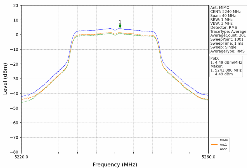
802.11n(HT20)_HCH_5240MHz_MIMO_NTNV
