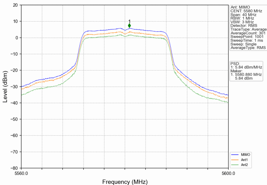
802.11a_MCH_5580MHz_MIMO_NTNV
