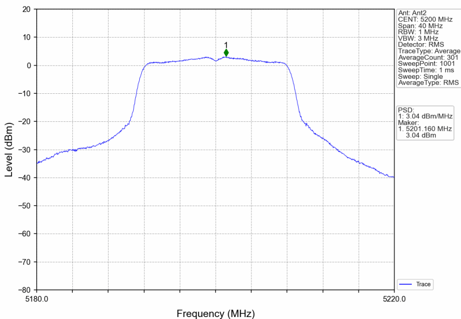
802.11a_MCH_5200MHz_MIMO_NTNV
