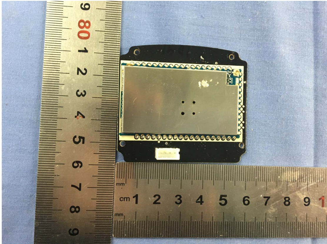
WIFI Module
