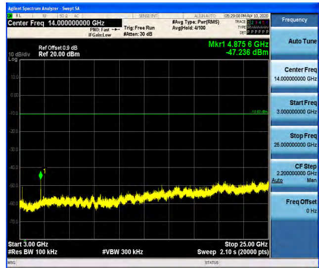
3GHz-25GHz
