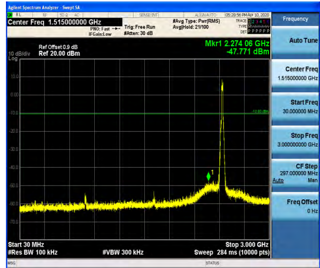
30MHz-3GHz
