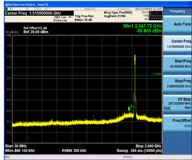
30MHz-3GHz
