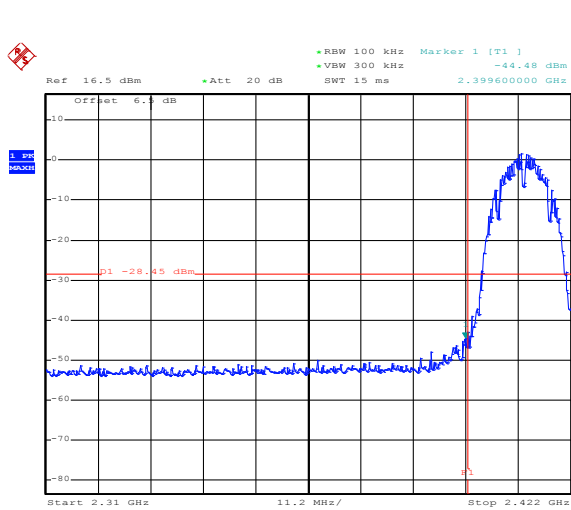
802.11b
