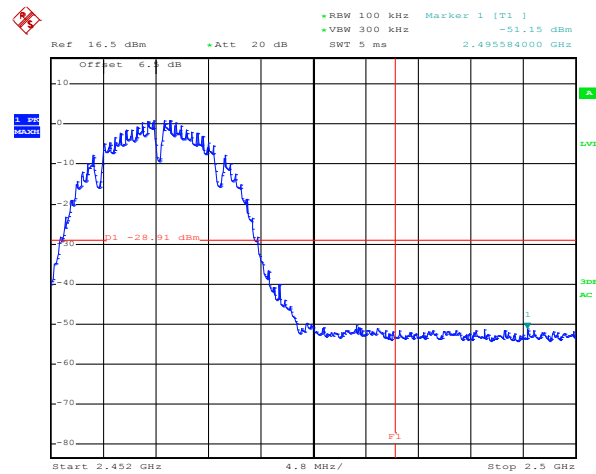
802.11b
