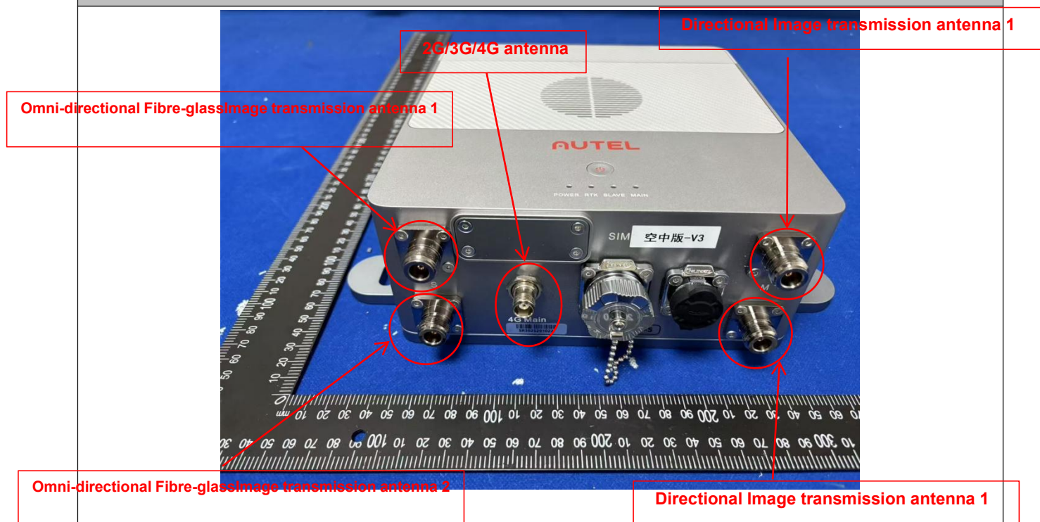
EUT Photo
