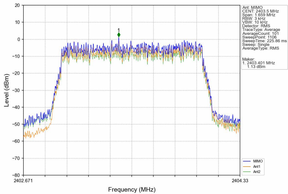
16QAM_LCH_2403.5MHz_MIMO_NTNV
