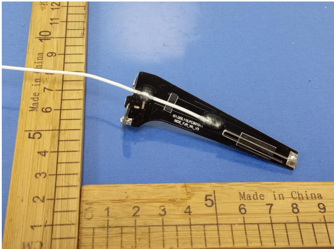
SRD FJL TRX ANT(ANT4)
