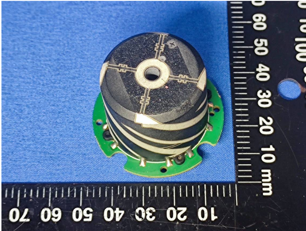
GPS Antenna 2
