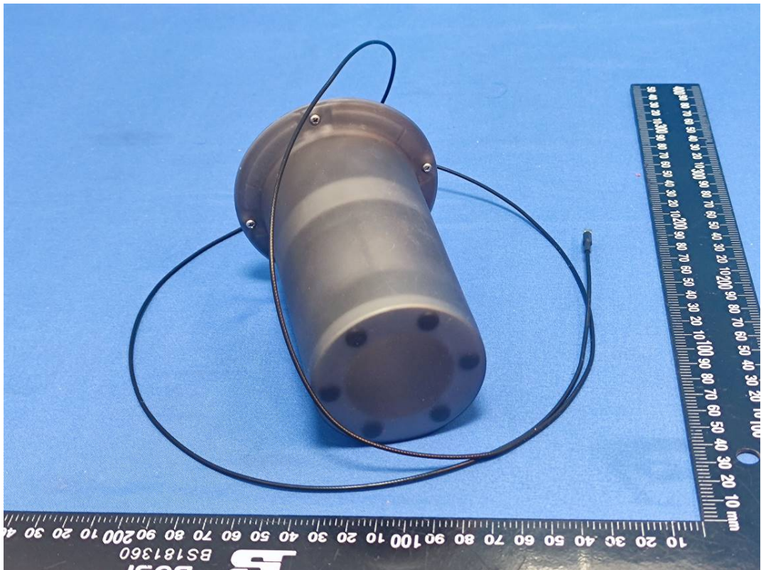
SRD Antenna-L(Chain 0)
