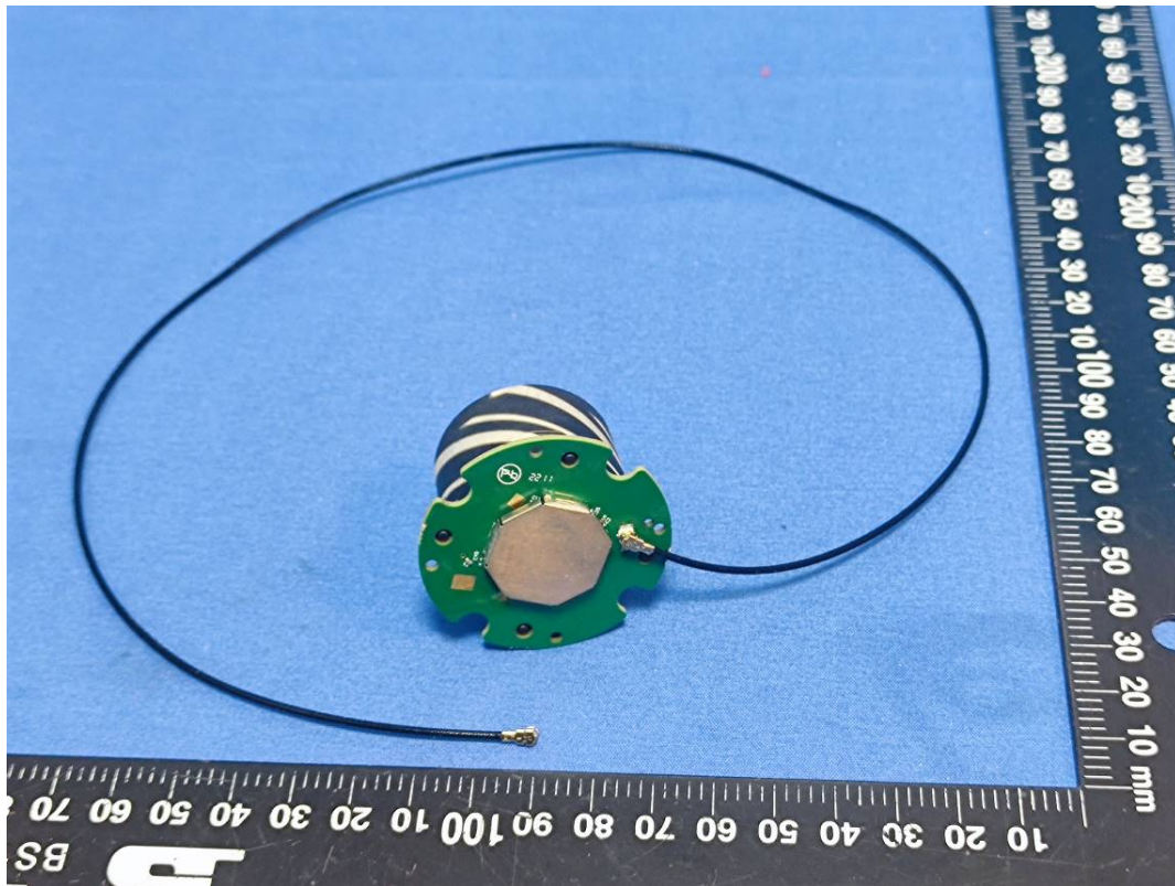
GPS Antenna 1
