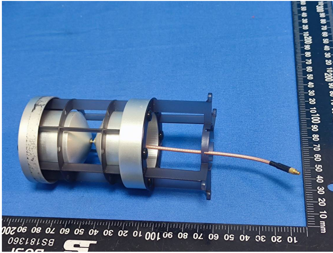
GPS Antenna 1
