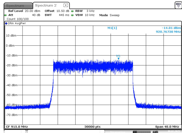
20M_915MHz_Chain 0
