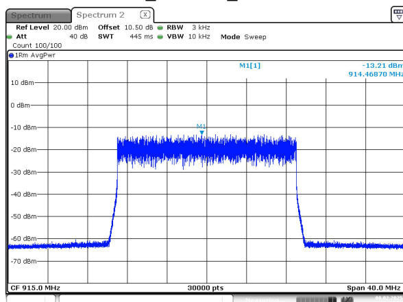
20M_915MHz_Chain 1
