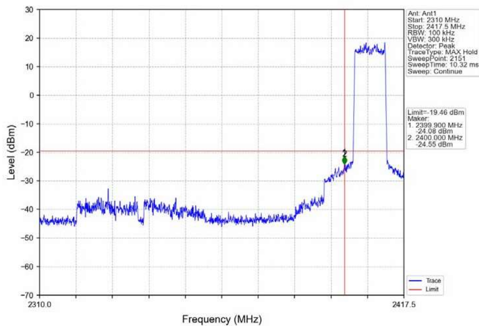
QPSK 10MHz_LCH_2407.5MHz_Ant1_NTNV
