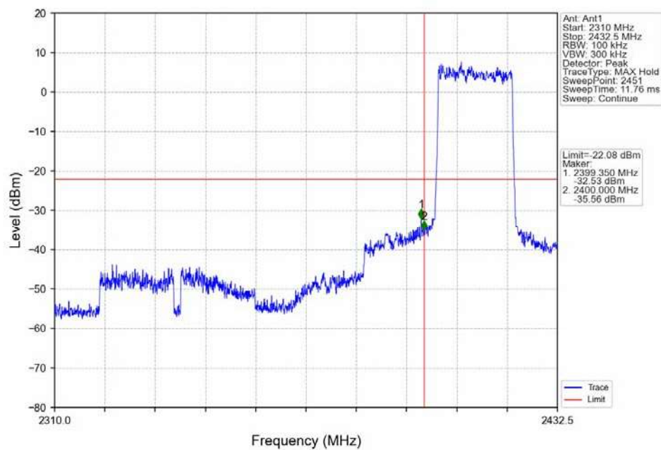
QPSK 20MHz_LCH_2412.5MHz_Ant1_NTNV
