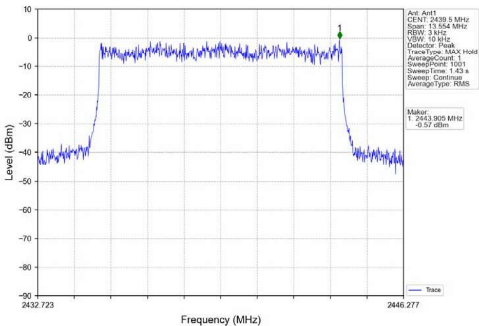
QPSK 10MHz_MCH_2439.5MHz_Ant1_NTNV
