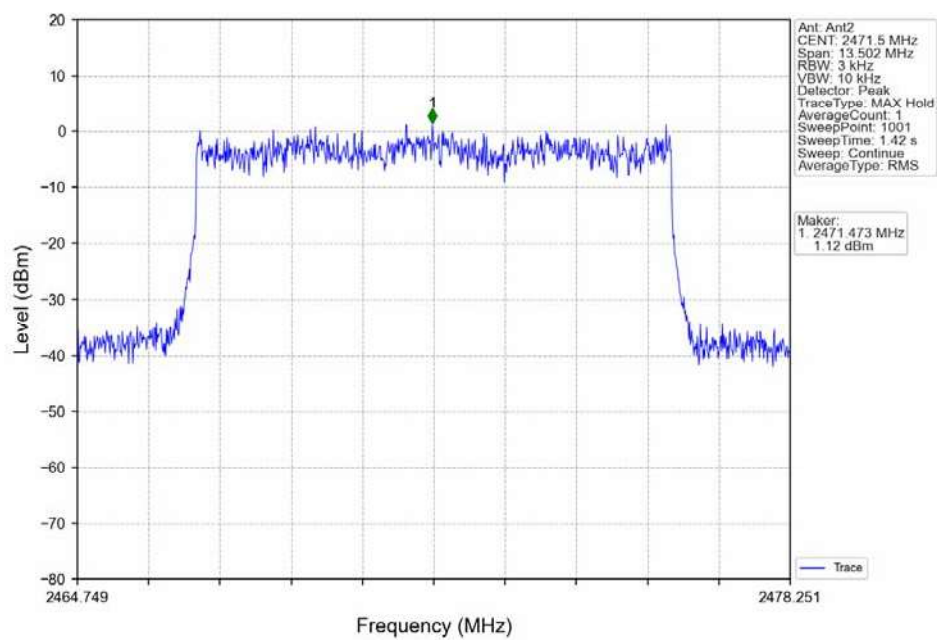
QPSK 10MHz_HCH_2471.5MHz_Ant2_NTNV
