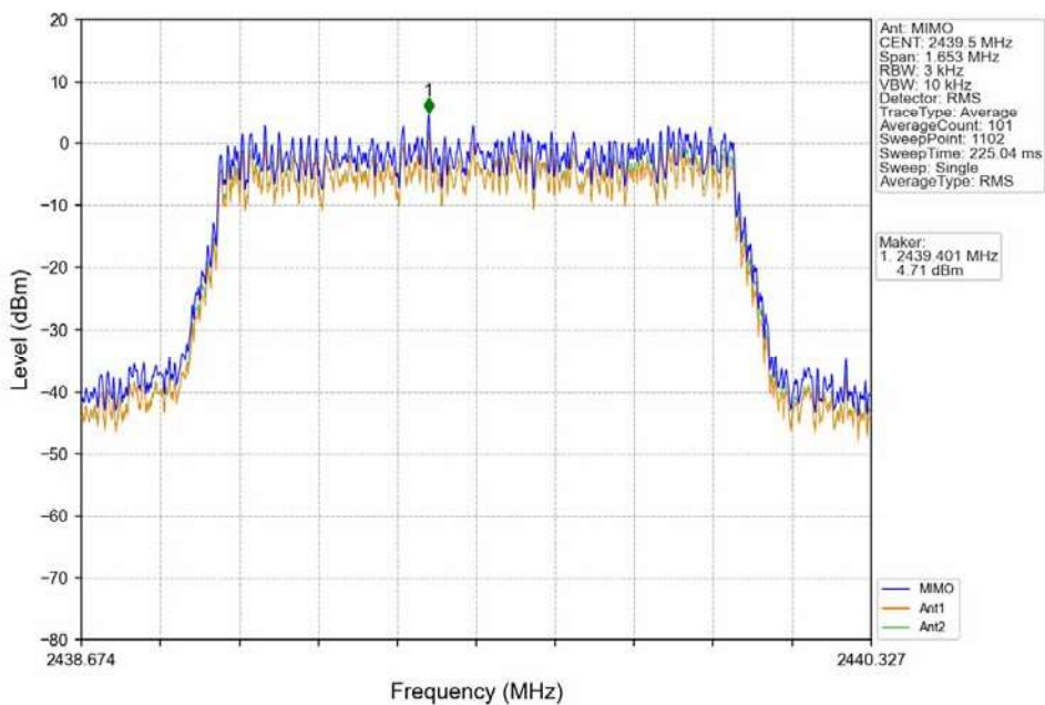
QPSK 1.4MHz_MCH_2439.5MHz_MIMO_NTNV
