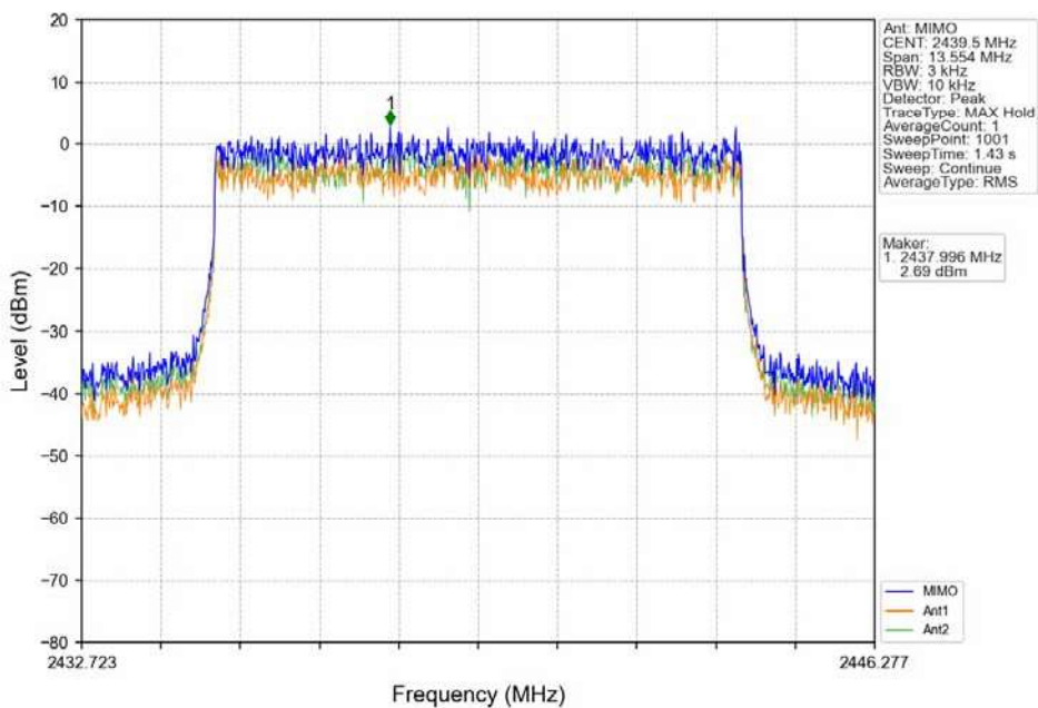
QPSK 10MHz_MCH_2439.5MHz_MIMO_NTNV
