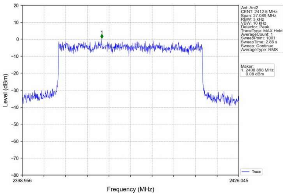
QPSK 20MHz_LCH_2412.5MHz_Ant2_NTNV
