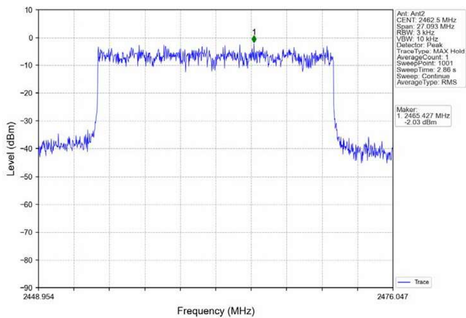
QPSK 20MHz_HCH_2462.5MHz_Ant2_NTNV
