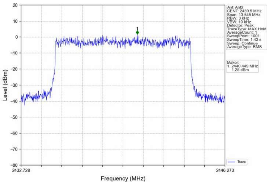
16QAM 10MHz_MCH_2439.5MHz_Ant2_NTNV
