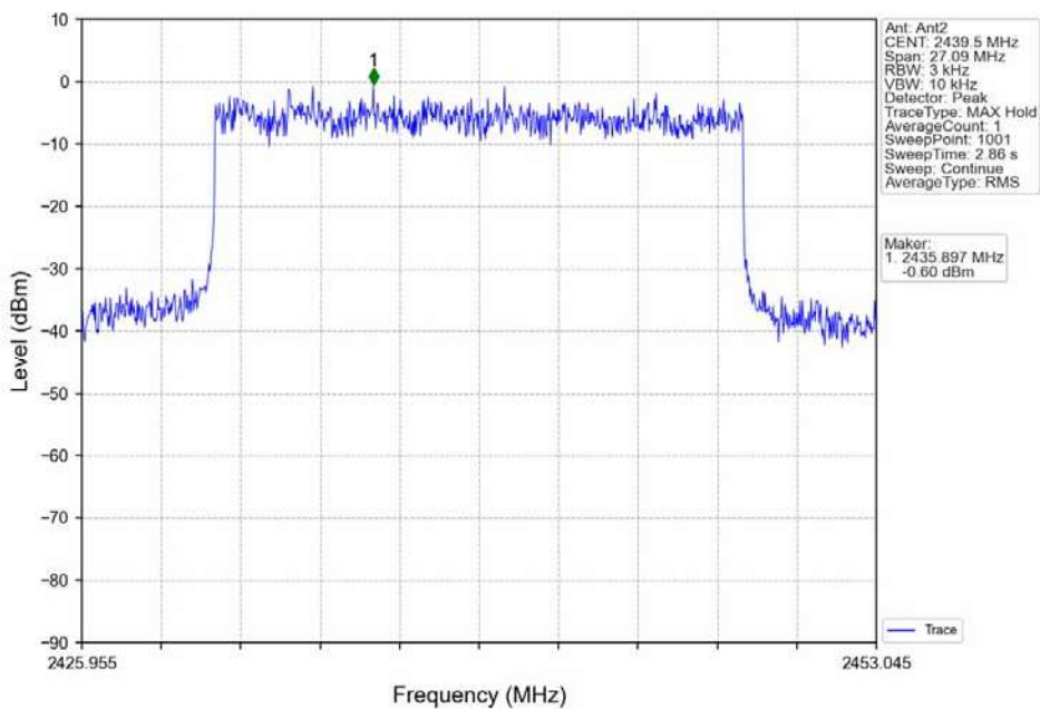
QPSK 20MHz_MCH_2439.5MHz_MIMO_NTNV
