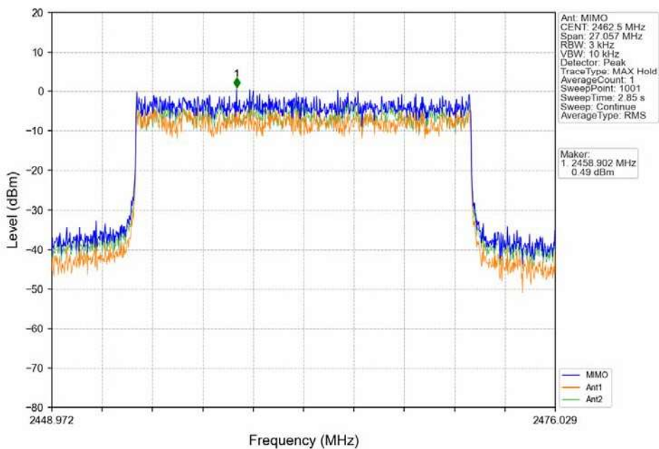
16QAM 20MHz_HCH_2462.5MHz_MIMO_NTNV
