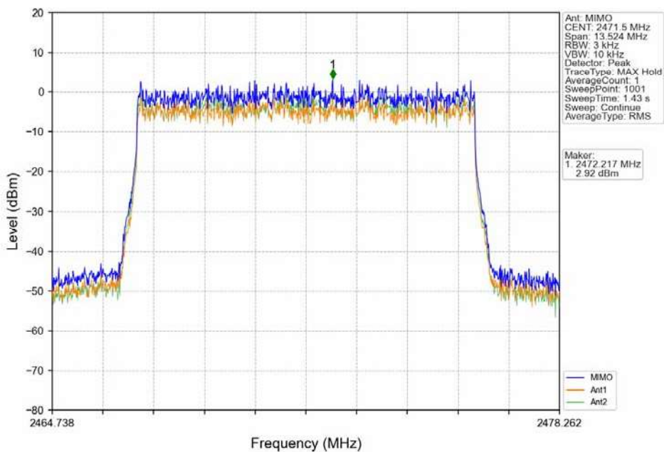
16QAM 10MHz_HCH_2471.5MHz_MIMO_NTNV
