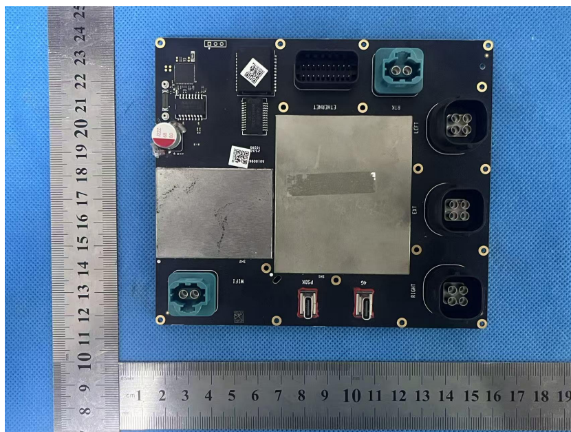
EUT Photo
