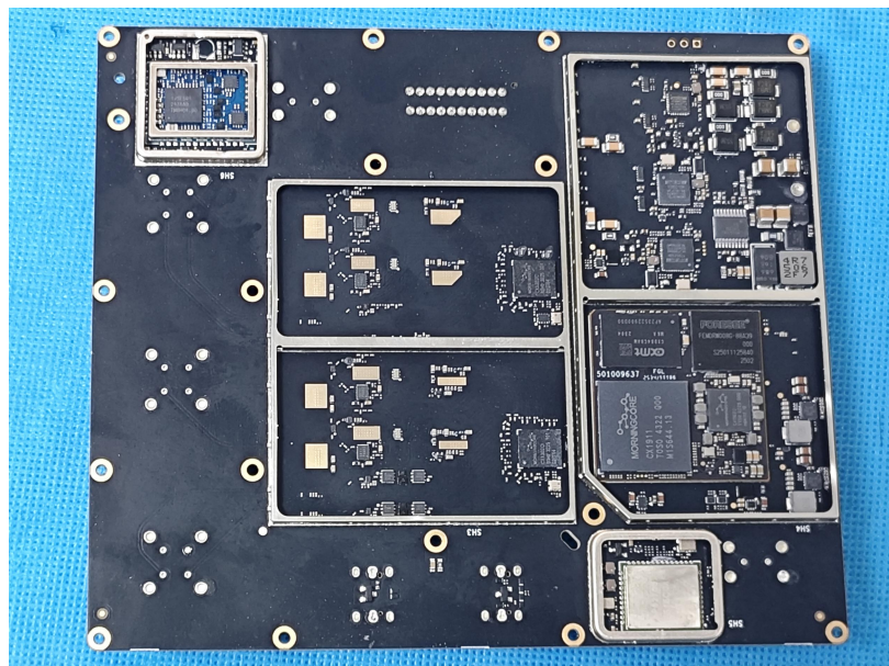
EUT Photo
