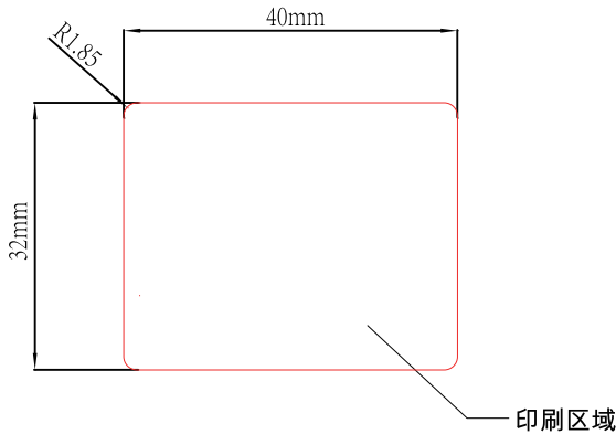
刀模图
