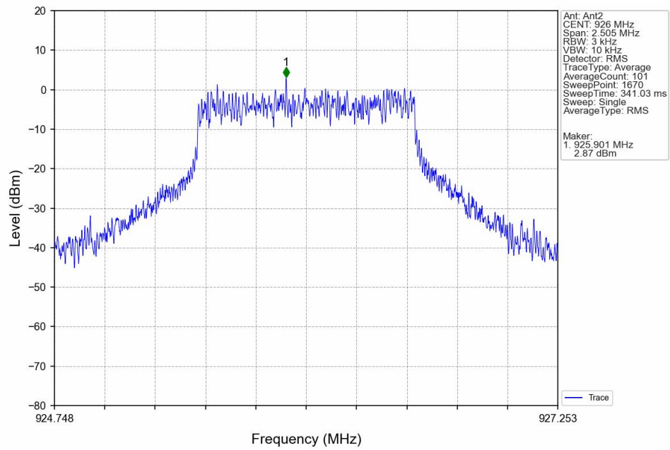
16QAM_HCH_926MHz_MIMO_NTNV
