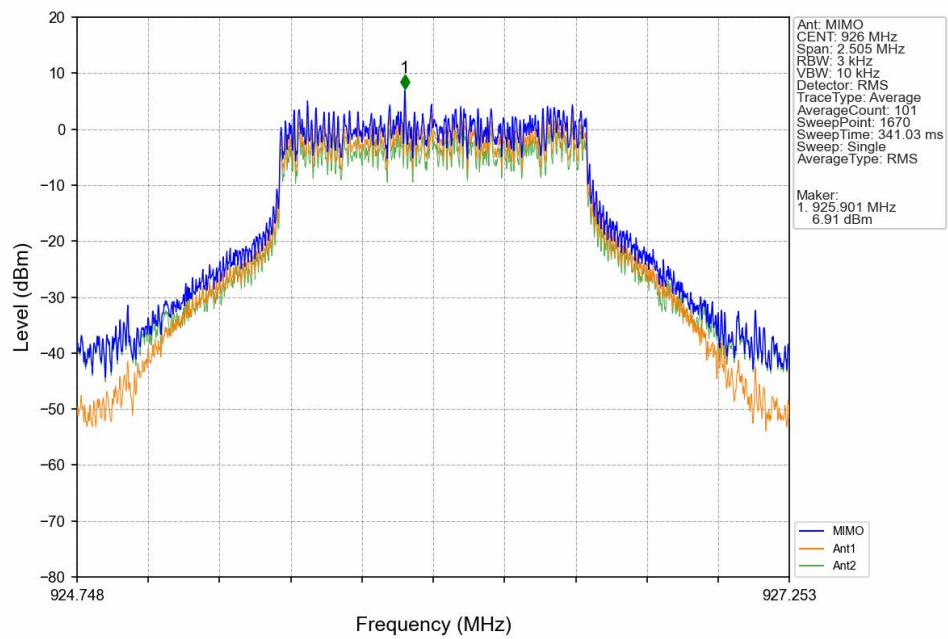
16QAM_HCH_926MHz_MIMO_NTNV
