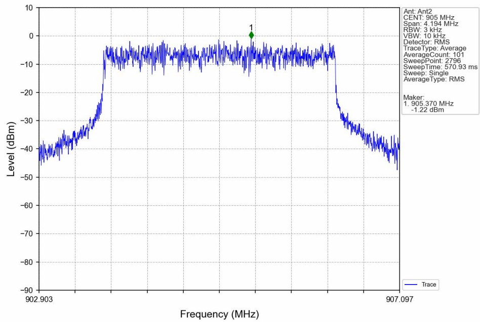
16QAM_LCH_905MHz_MIMO_NTNV
