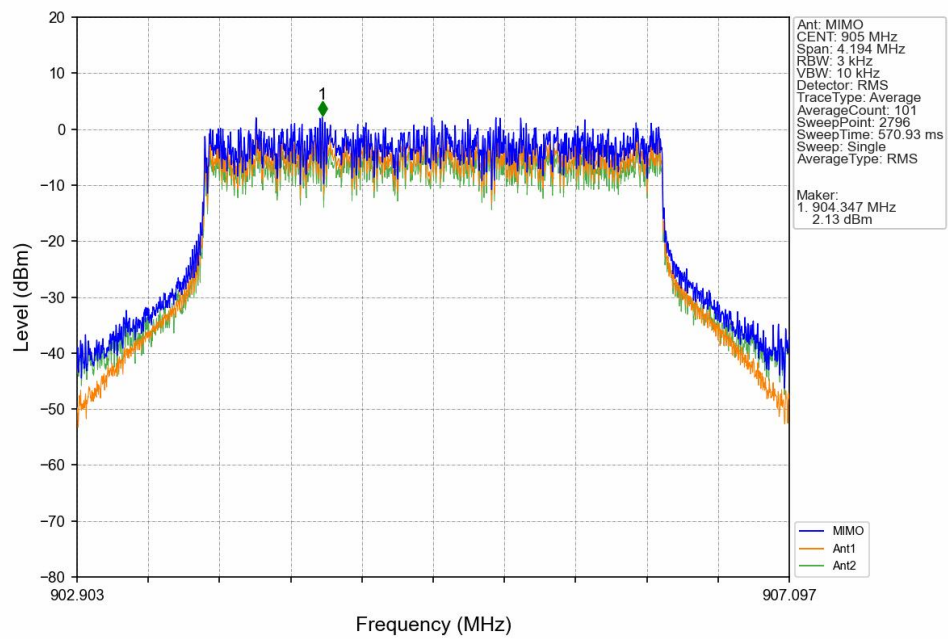
16QAM_LCH_905MHz_MIMO_NTNV
