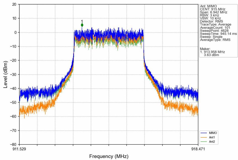
QPSK_MCH_915MHz_MIMO_NTNV
