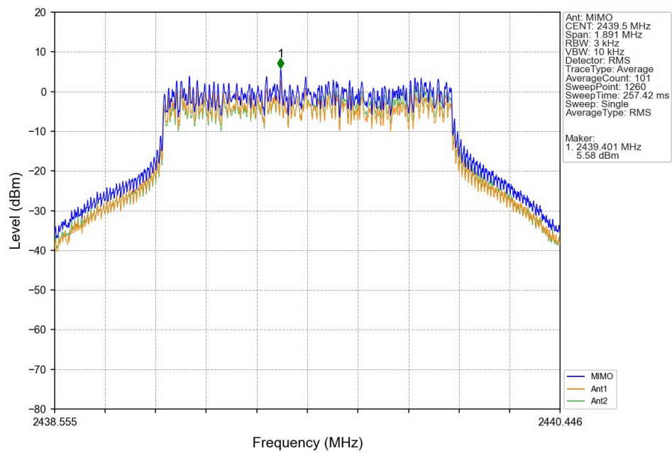
QPSK_MCH_2439.5MHz_MIMO_NTNV
