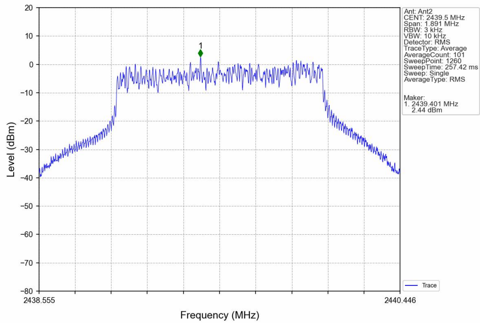
QPSK_MCH_2439.5MHz_MIMO_NTNV
