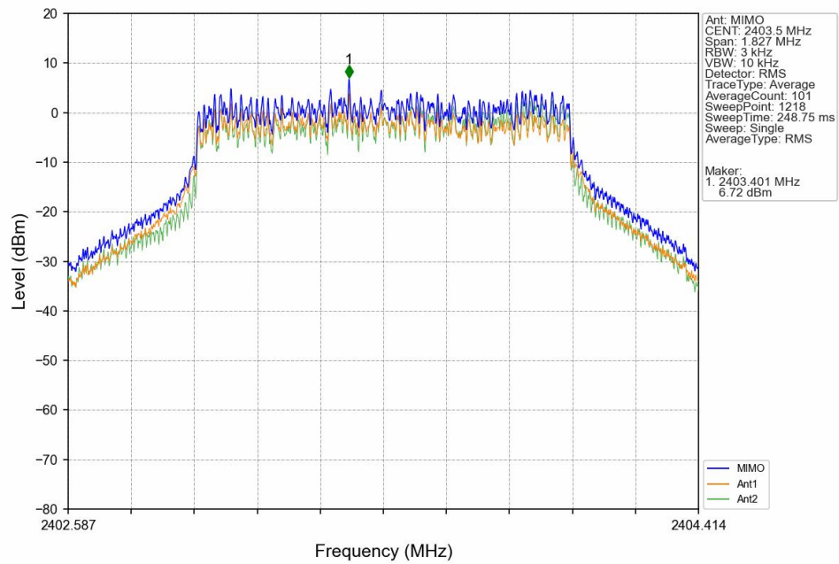
16QAM_LCH_2403.5MHz_MIMO_NTNV
