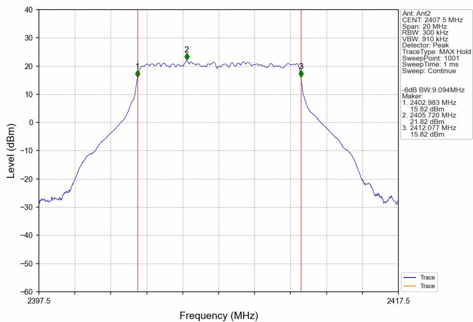
QPSK_LCH_2407.5MHz_Ant2_NTNV
