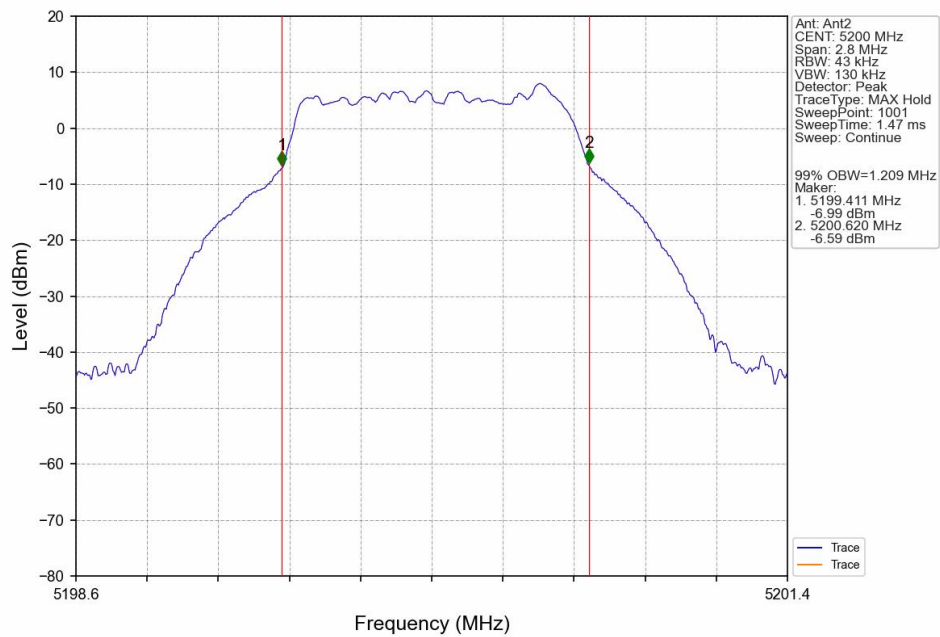
16QAM_MCH_5200MHz_Ant2_NTNV
