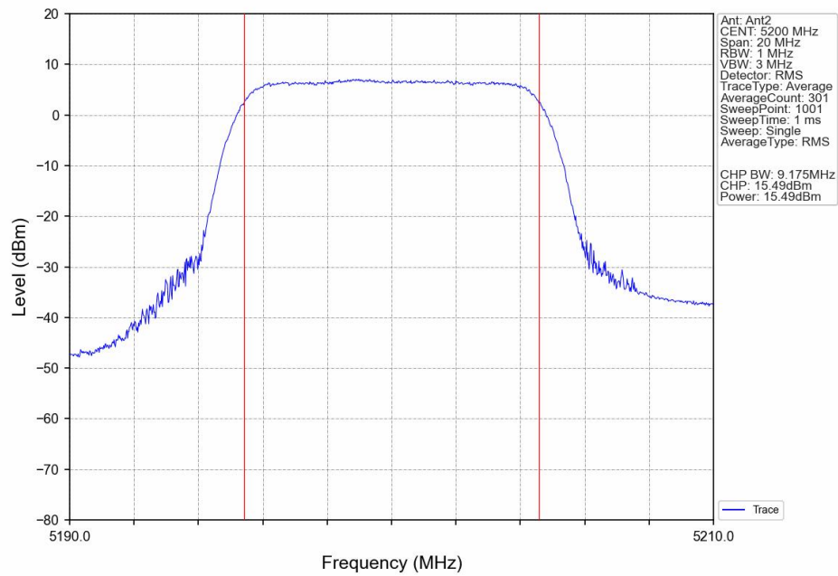
QPSK_MCH_5200MHz_Ant2_NTNV
