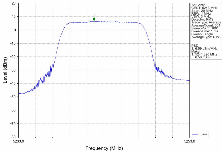
16QAM_HCH_5243MHz_MIMO_NTNV
