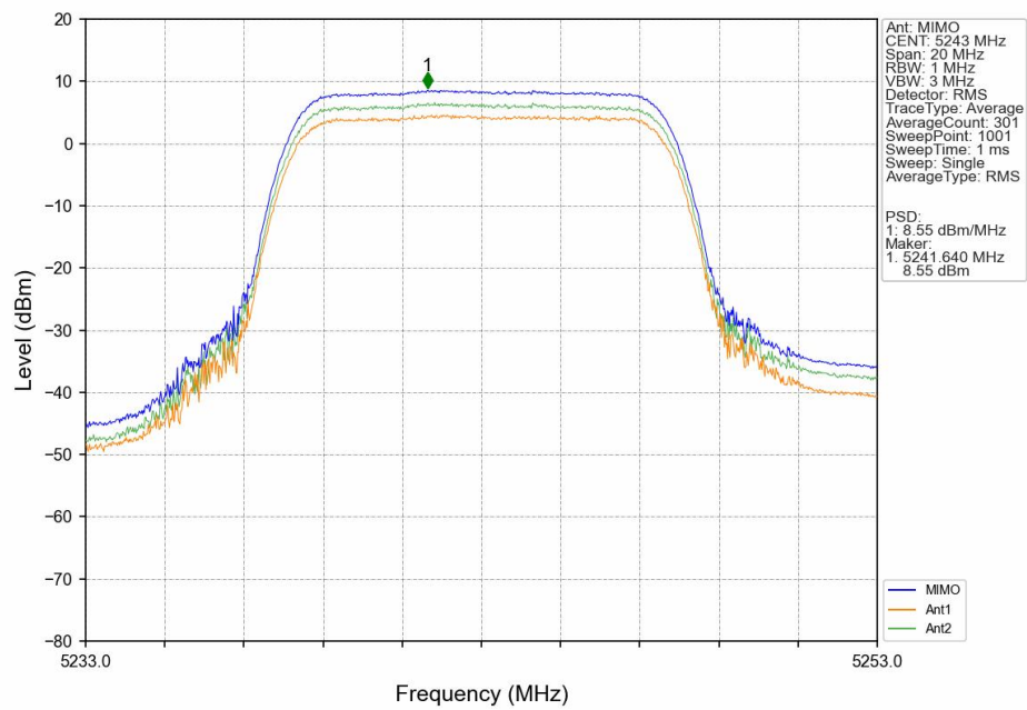
16QAM_HCH_5243MHz_MIMO_NTNV
