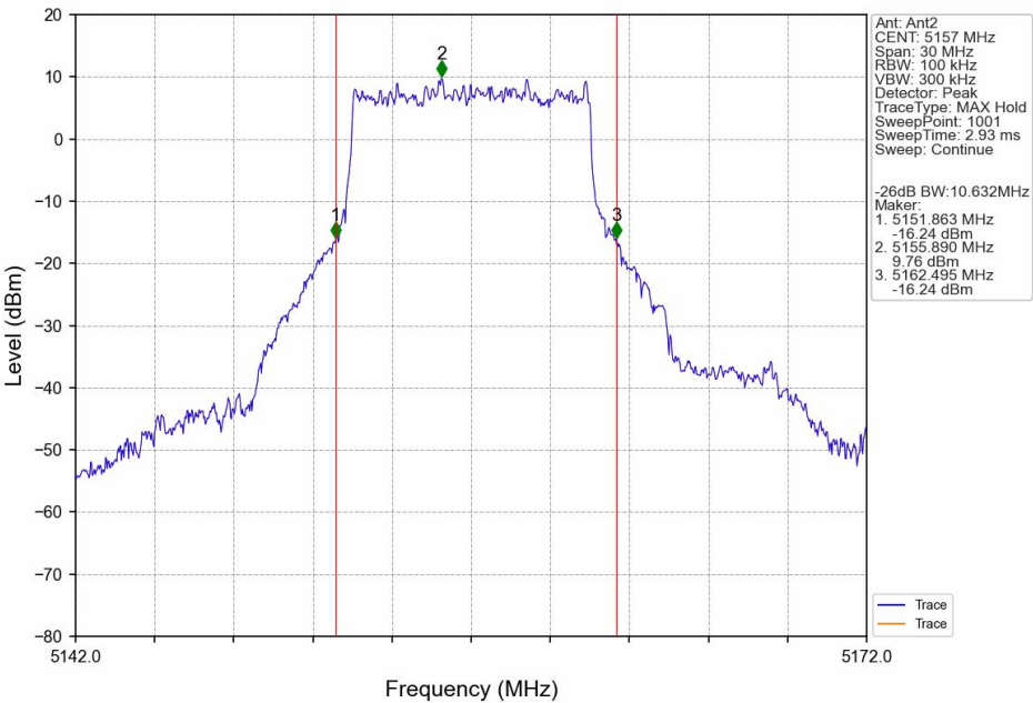
QPSK LCH 5157MHz_Ant2_NTNV
