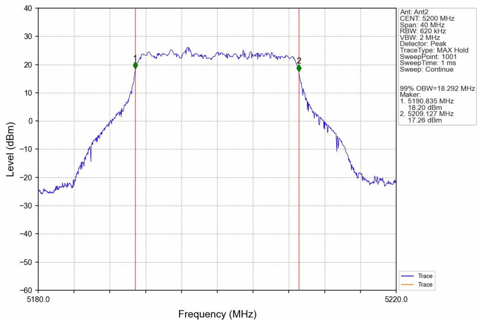
16QAM_MCH_5200MHz_Ant2_NTNV
