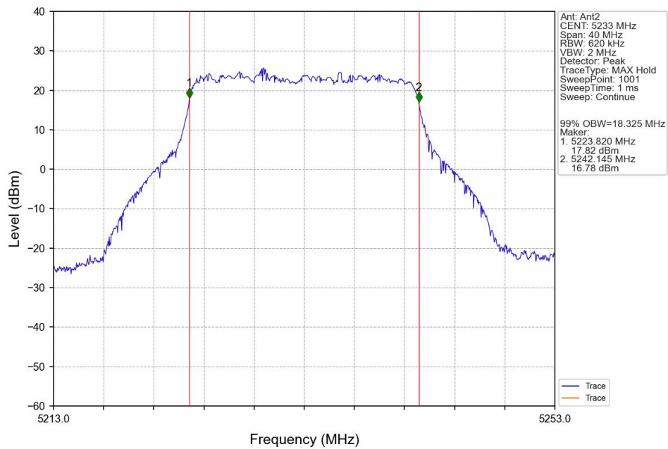
QPSK_HCH_5233MHz_Ant2_NTNV
