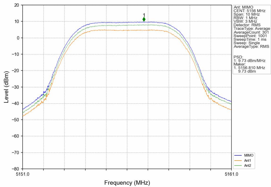
16QAM_LCH_5156MHz_MIMO_NTNV
