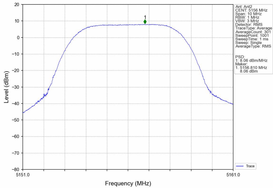
16QAM_LCH_5156MHz_MIMO_NTNV
