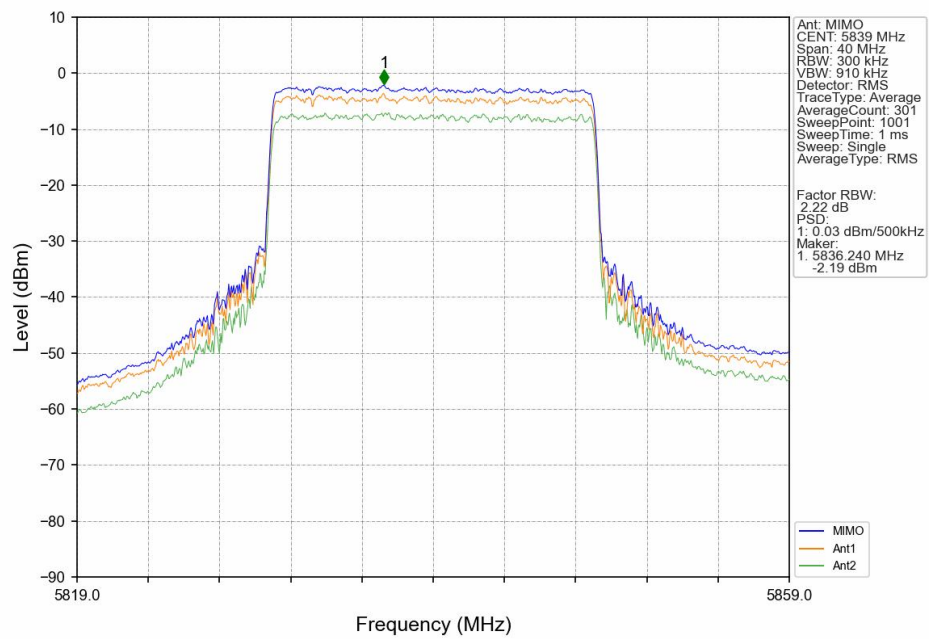
16QAM_HCH_5839MHz_MIMO_NTNV
