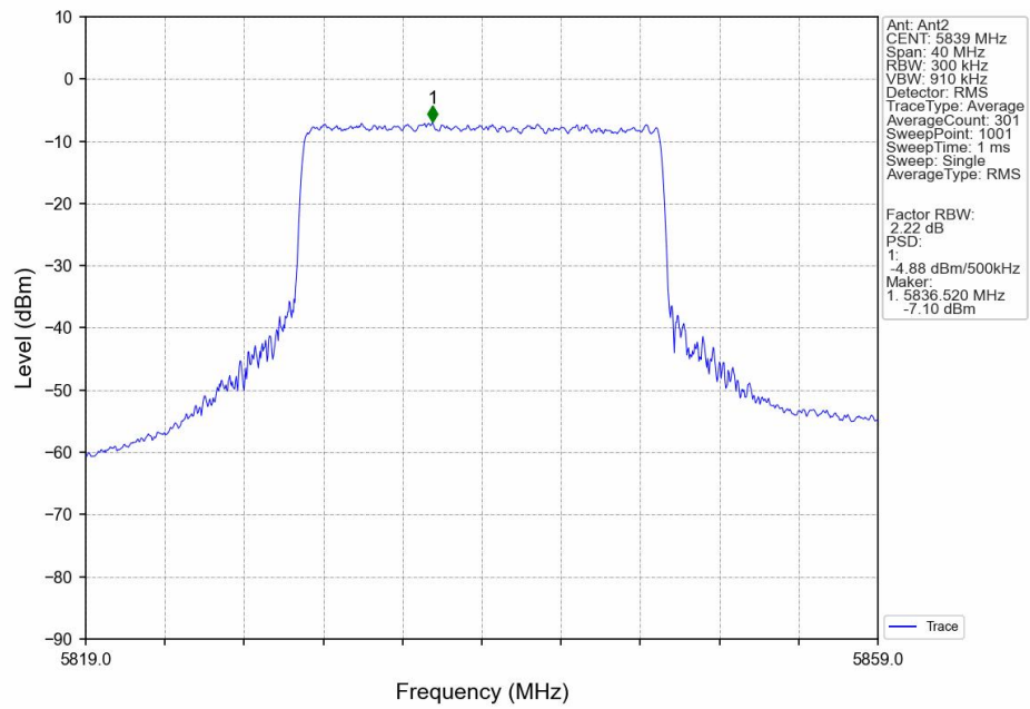
16QAM_HCH_5839MHz_MIMO_NTNV
