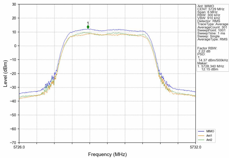
16QAM_LCH_5729MHz_MIMO_NTNV
