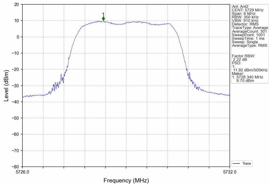
16QAM_LCH_5729MHz_MIMO_NTNV
