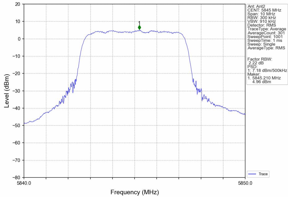
16QAM_HCH_5845MHz_MIMO_NTNV
