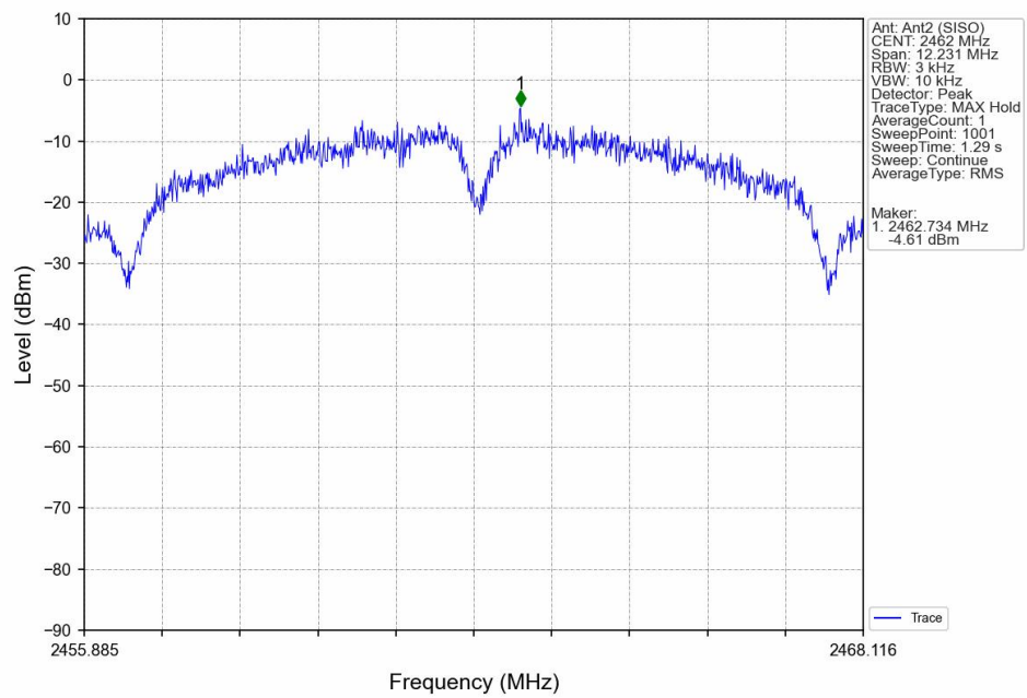
802.11b_HCH_2462MHz_Ant2 (SISO)_NTNV
