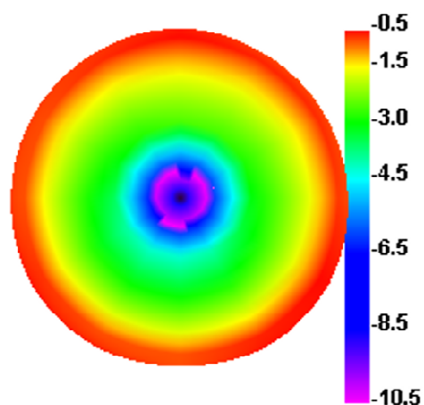
5150.000MHz E1
