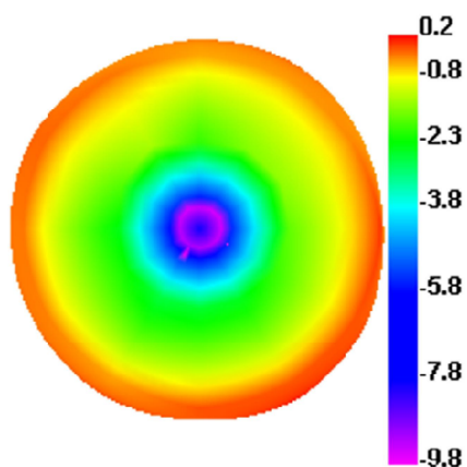
5850.000MHz
