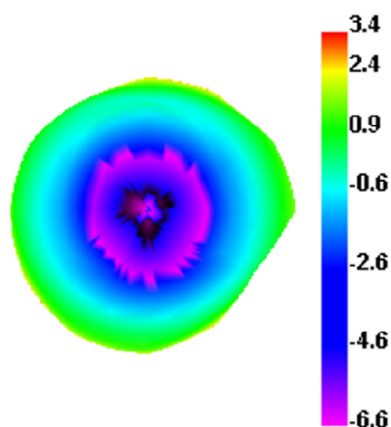
2450.000MHz E1
