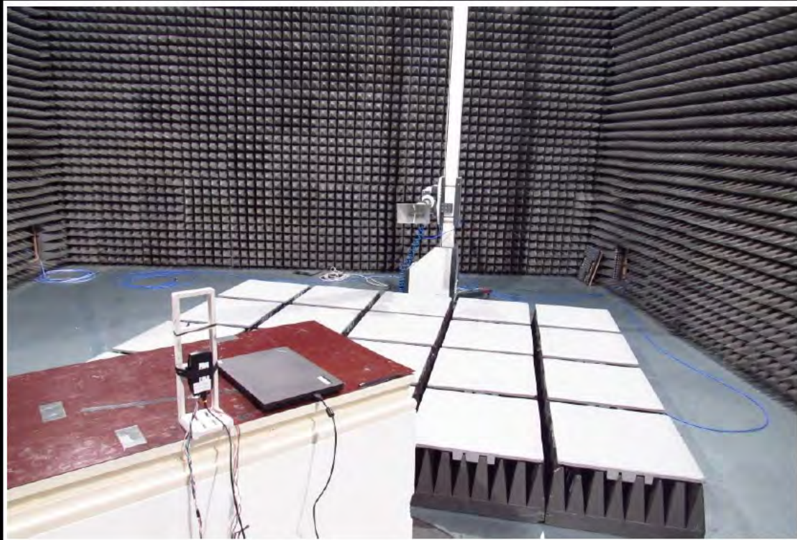
1-6.5GHz
