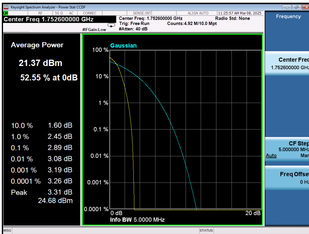
WCDMA Band4\H
