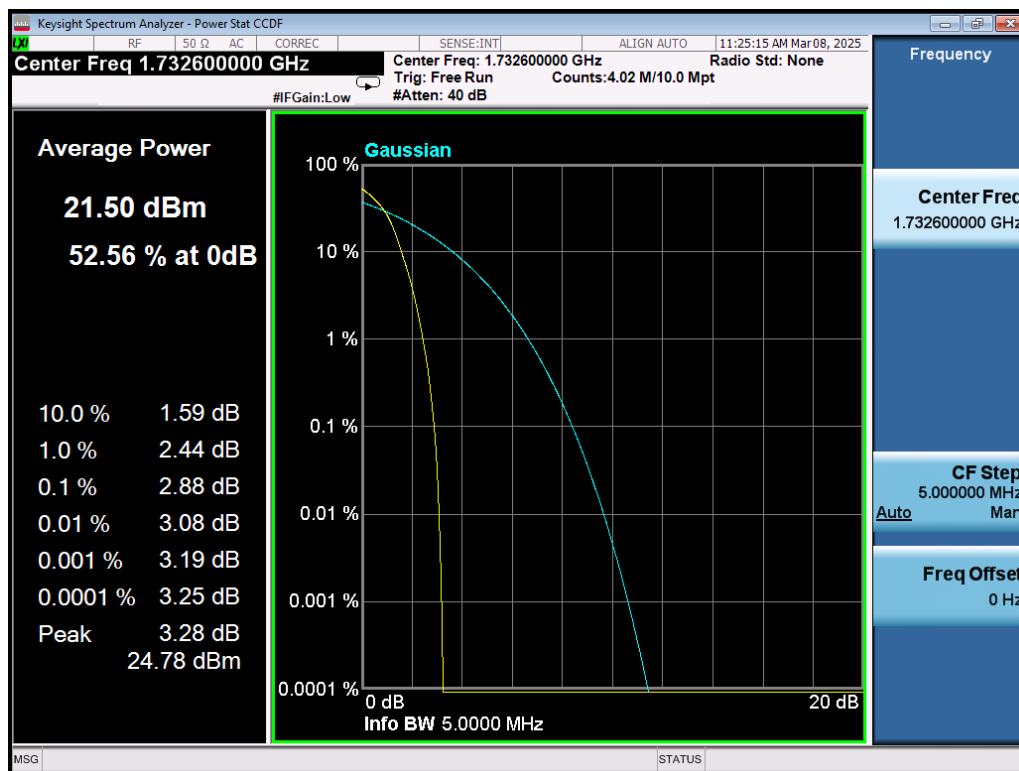
WCDMA Band4\M
