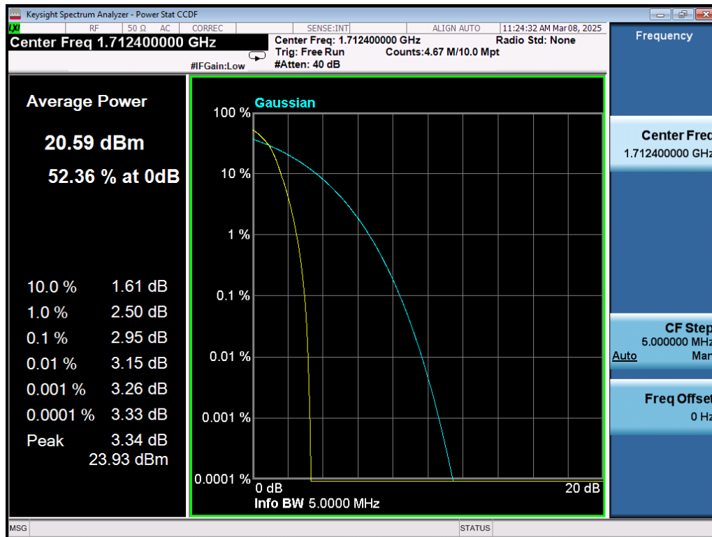
WCDMA Band4\L
