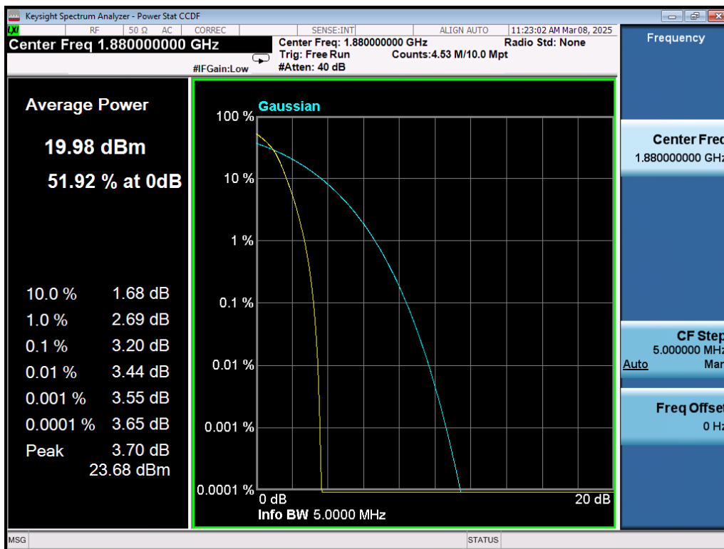
WCDMA Band2\M
