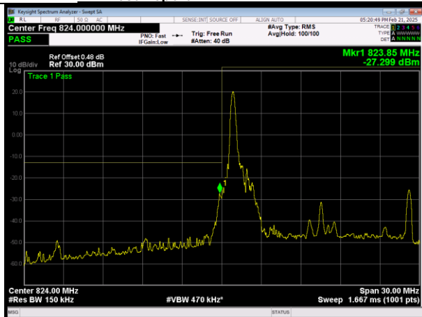
LLTE Band26 (824-849) QAM64 BW=15MHz Channel=26865 RB Size=1 Position=#0
