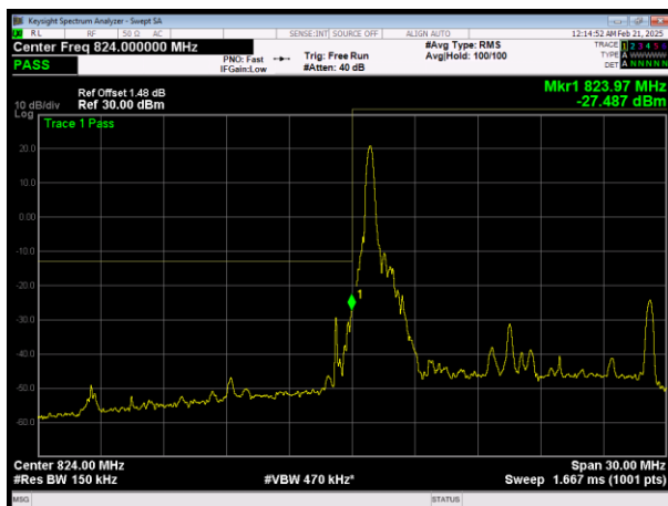
L\LTE Band26 (824-849) QPSK BW=15MHz Channel=26865 RB Size=1 Position=#0
