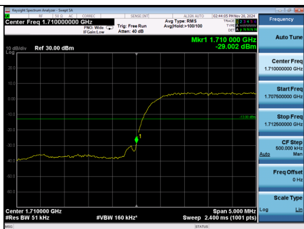
WCDMA B4/L
