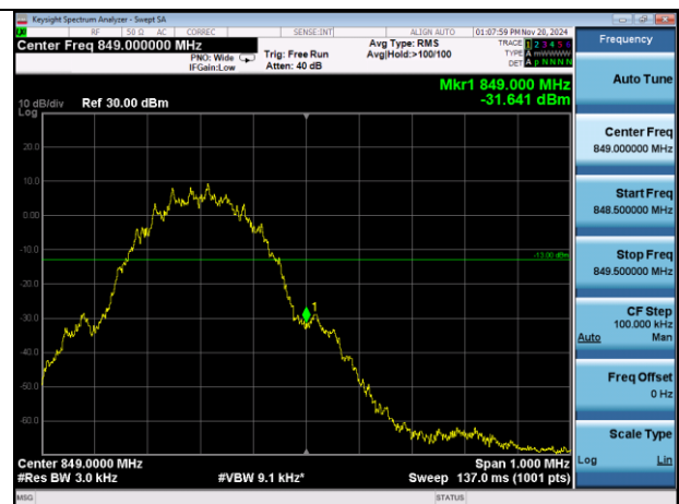
EGPRS850\H
