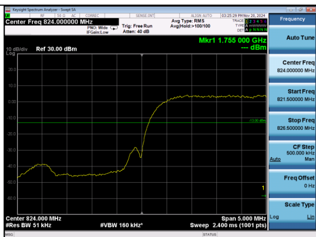
WCDMA B5/L
