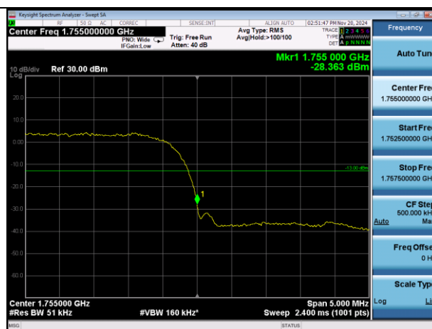
WCDMA B4/H
