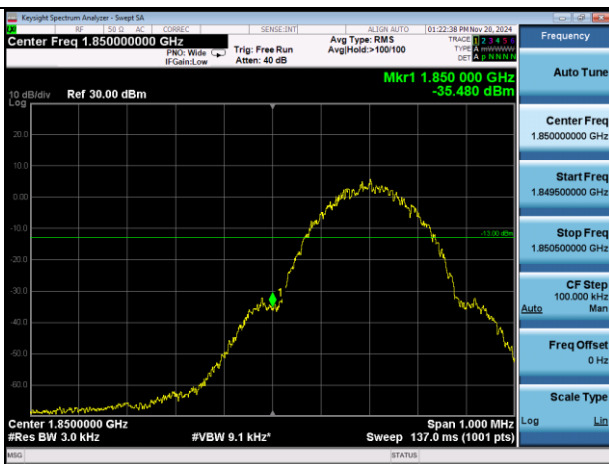
GPRS1900L
