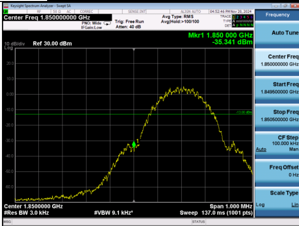
GSM1900L
