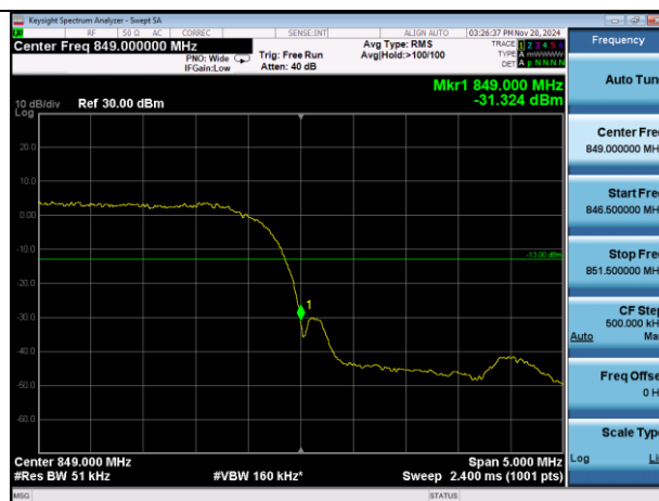
WCDMA B5/H
