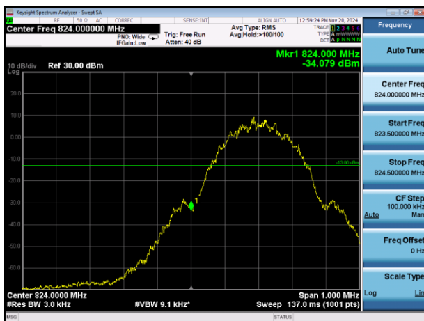
GPRS850\L
