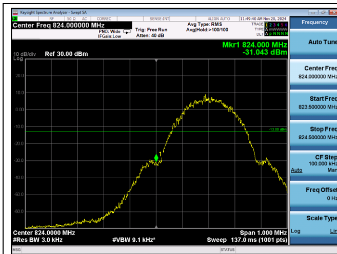
GSM850\L
