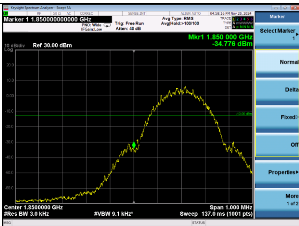
EGPRS1900L
