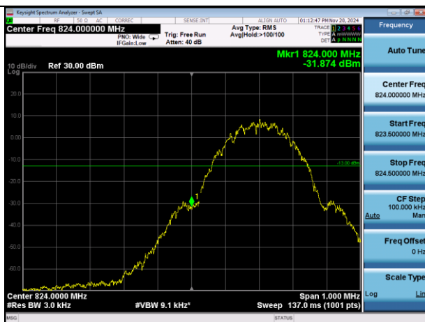
EGPRS850\L
