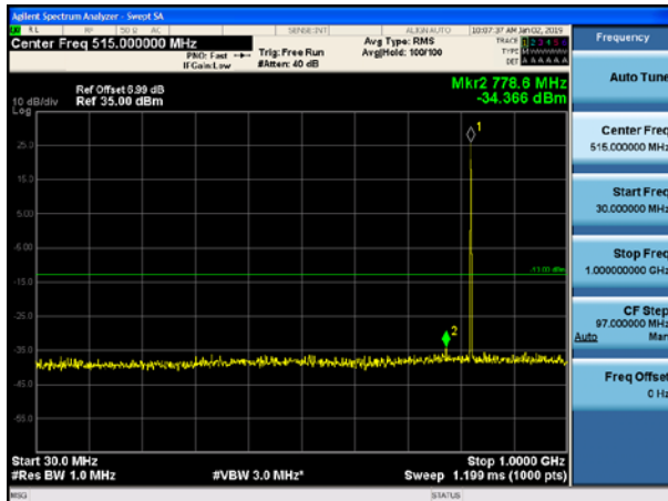
GSM 850-LCH-GSM
