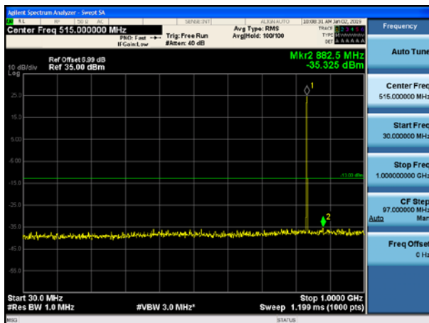
GSM 850-MCH-GSM
