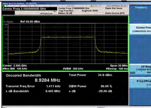
Band38 10MHz QPSK 38000 50RB#0
