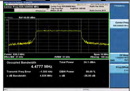
Band5 5MHz 16QAM 20425 25RB#0
