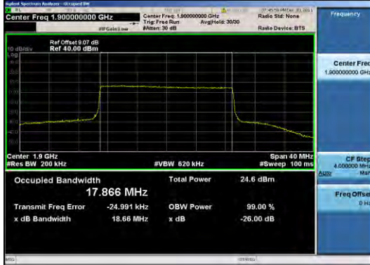
Band2 20MHz QPSK 19100 100RB#0
