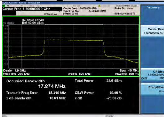
Band2 20MHz 16QAM 19100 100RB#0
