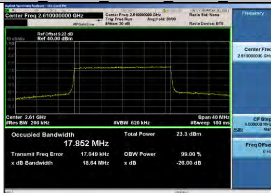
Band38 20MHz 16QAM 38150 100RB#0
