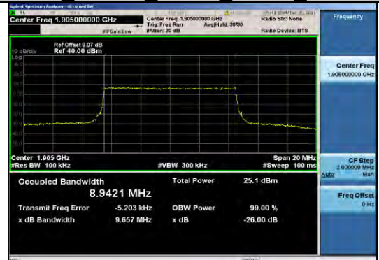
Band2 10MHz QPSK 19150 50RB#0
