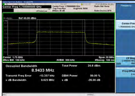
Band4 10MHz QPSK 20350 50RB#0
