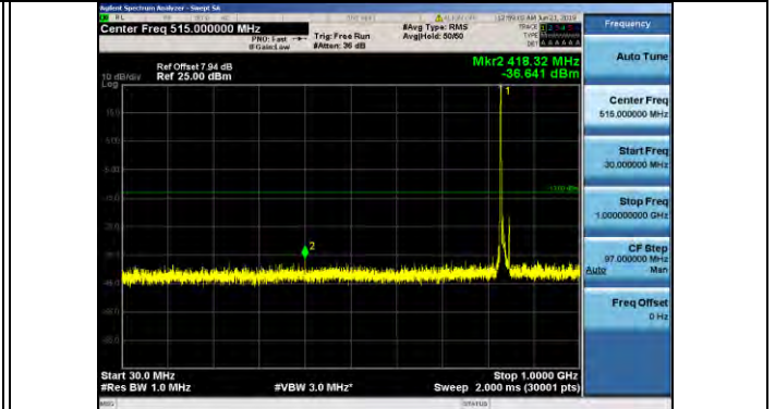
Band5 10MHz 16QAM 20525 1RB#0
