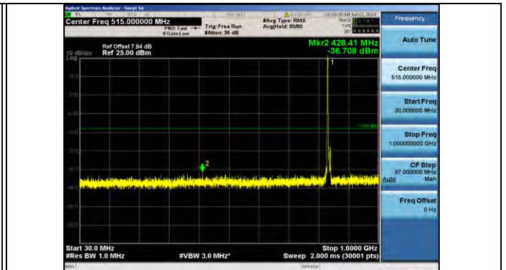
Band5 5MHz QPSK 20525 1RB#0
