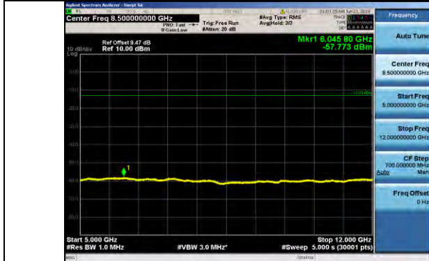
Band5 10MHz QPSK 20600 1RB#0
