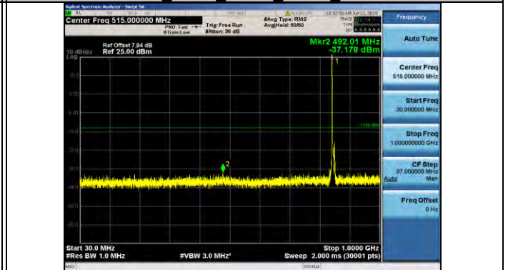
Band5 5MHz QPSK 20625 1RB#0
