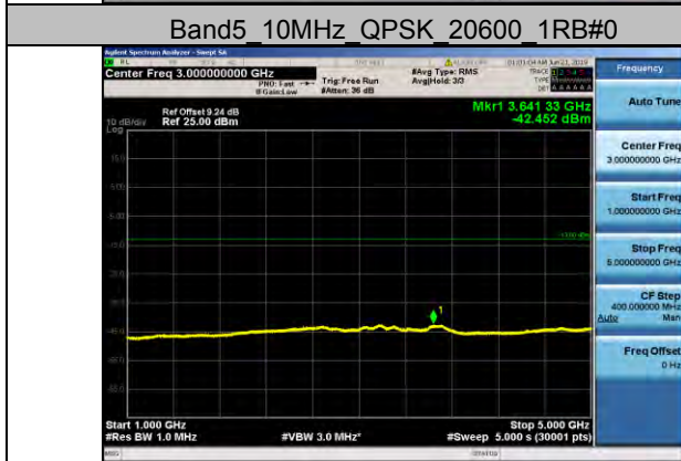
Band5 10MHz QPSK 20600 1RB#0
