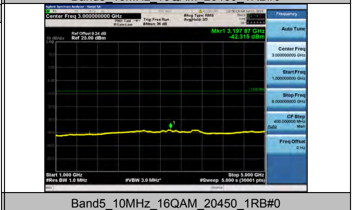
Band5 10MHz 16QAM 20450 1RB#0
