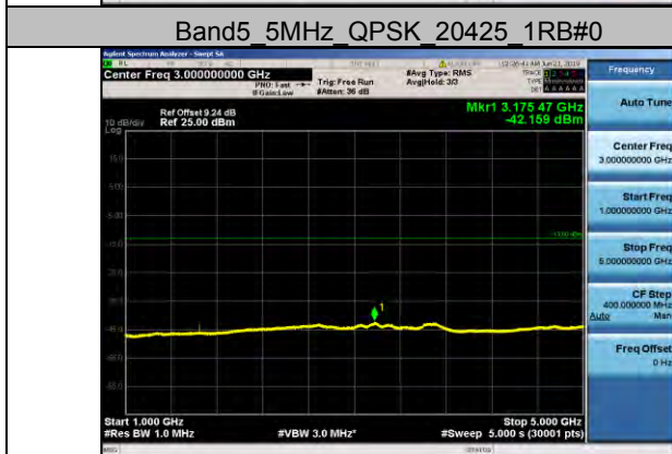
Band5 5MHz QPSK 20425 1RB#0
