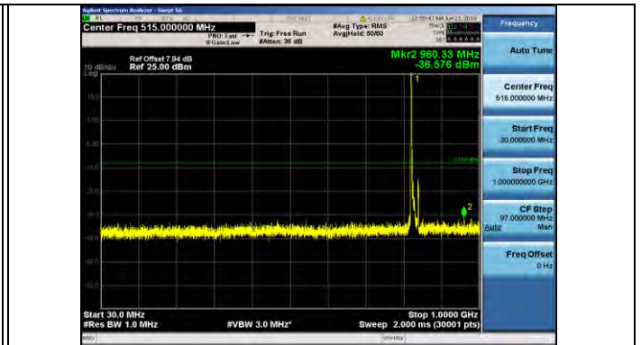
Band5 10MHz 16QAM 20450 1RB#0
