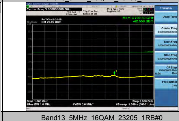
Band13 5MHz 16QAM 23205 1RB#0
