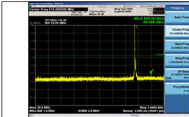
Band13 10MHz 16QAM 23230 1RB#0
