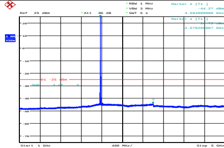
Band38-5MHz-QPSK-37775-1RB#0-Range4:1000~5000MHz
