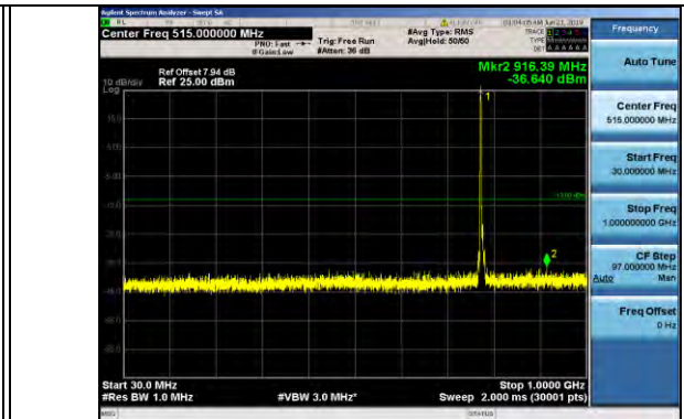
Band13 5MHz 16QAM 23205 1RB#0
