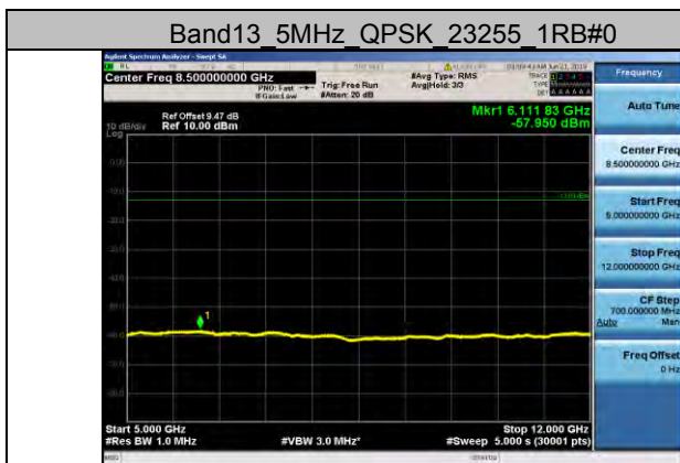
Band13 5MHz QPSK 23255 1RB#0
