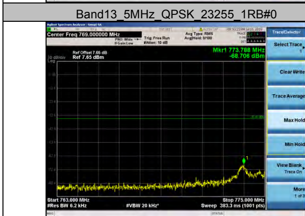
Band13 5MHz QPSK 23255 1RB#0
