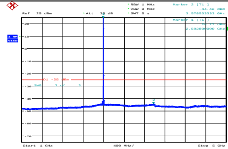
Band38-5MHz-QPSK-38000-1RB#0-Range4:1000~5000MHz
