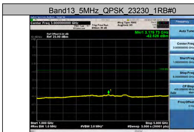
Band13 5MHz QPSK 23230 1RB#0
