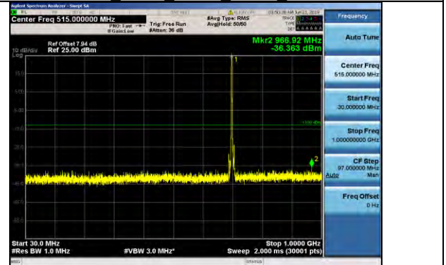
Band17 5MHz QPSK 23755 1RB#0
