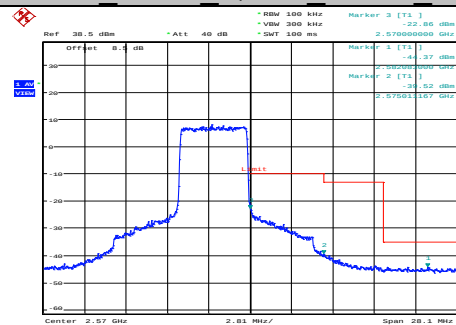
Band7 5MHz QPSK 21425 25RB#0
