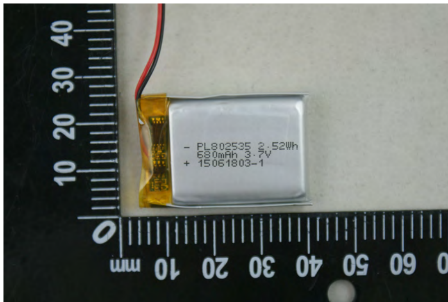
EUT Photo 12
