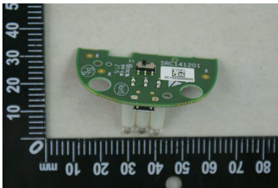
EUT Photo 14
