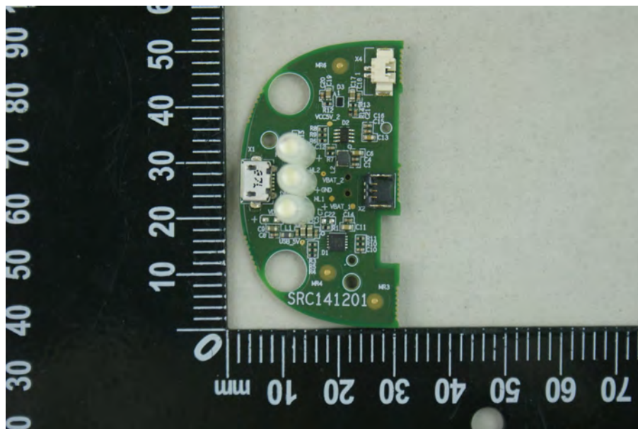
EUT Photo 13
