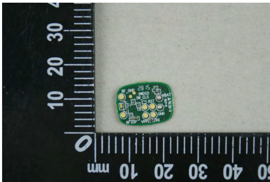
EUT Photo 8
