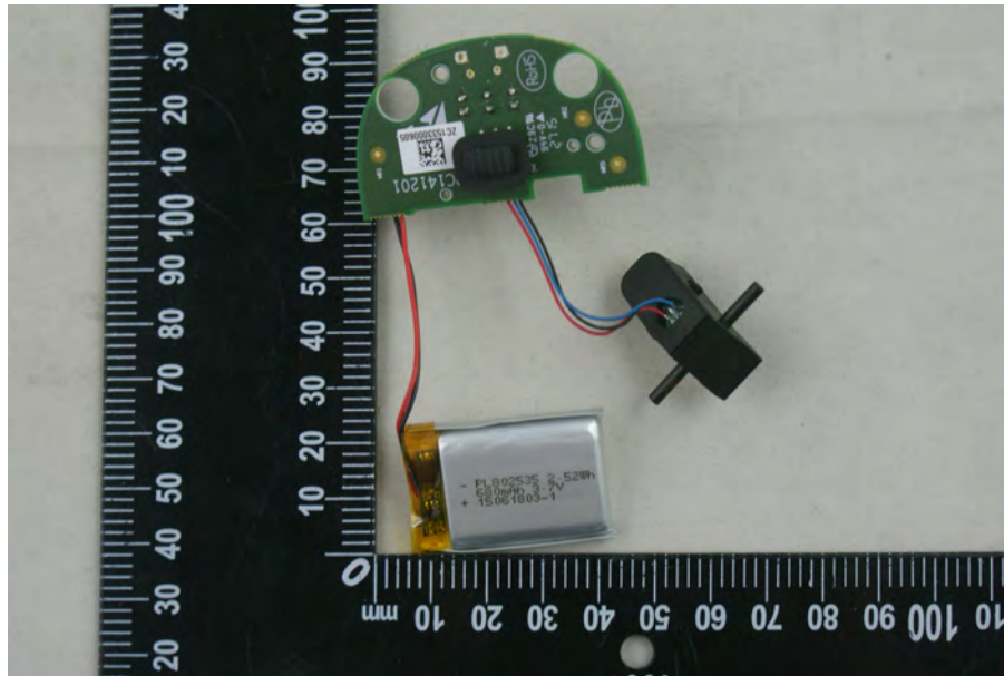
EUT Photo 11
