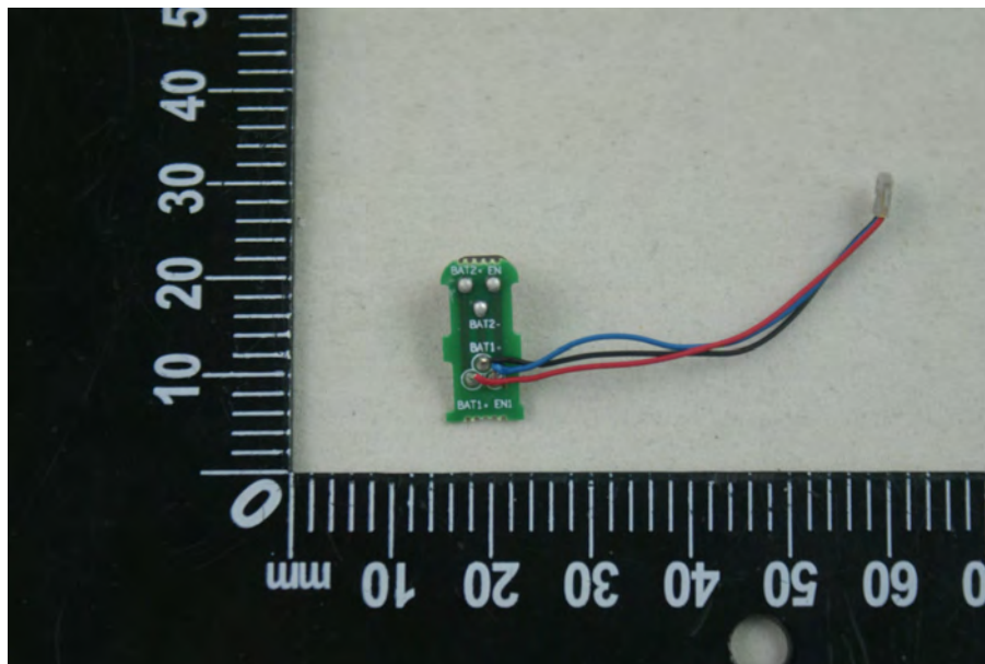
EUT Photo 16
