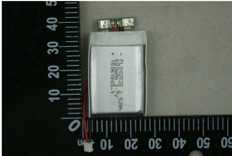
EUT Photo 17
