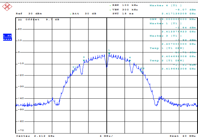
802.11b
