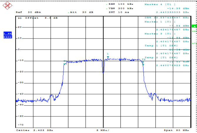
802.11n(HT40)
