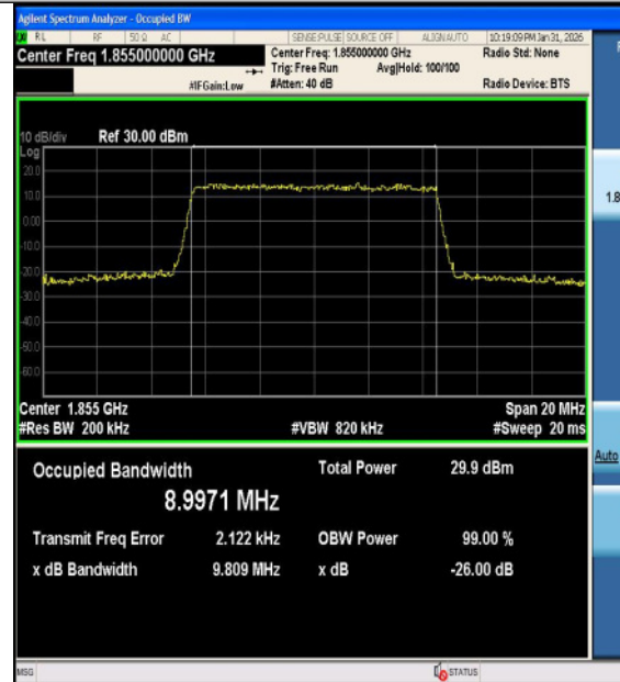
Band2-10MHz-16QAM-18900-50RB#0-PASS
