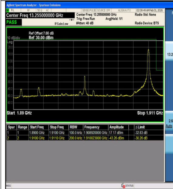
Band2-20MHz-16QAM-19100-1RB#99-PASS
