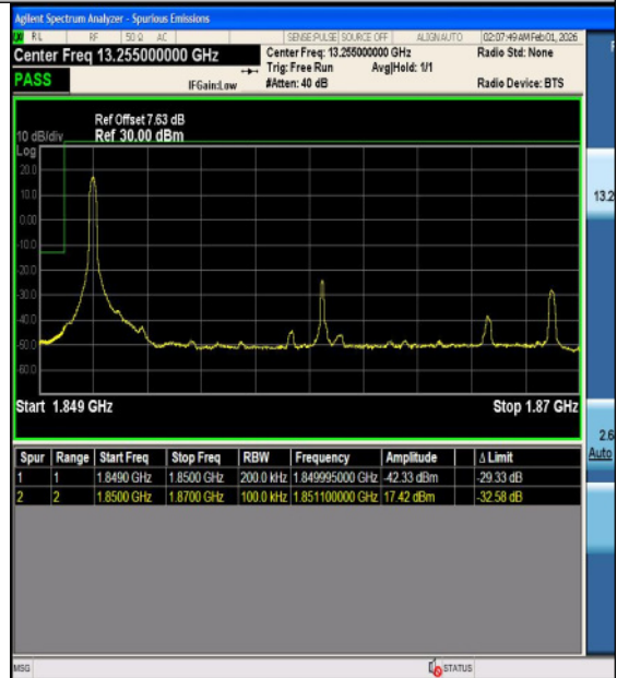
Band2-20MHz-16QAM-18700-100RB#0-PASS
