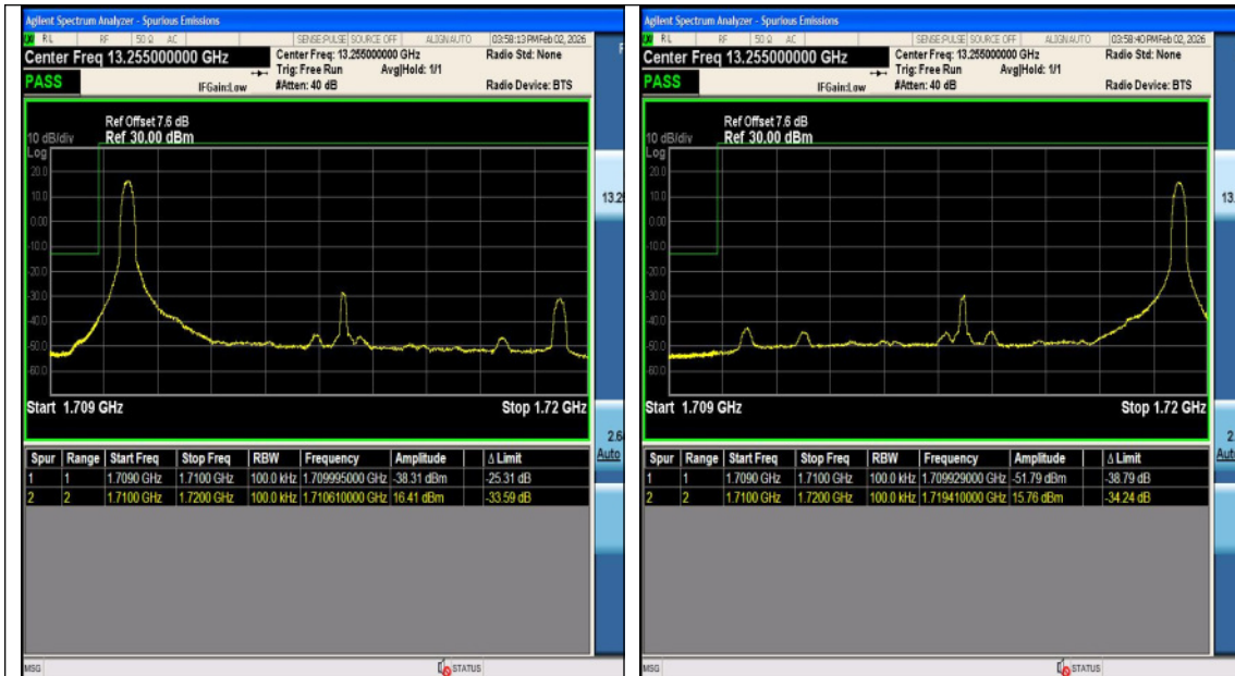
Band4-10MHz-QPSK-20000-50RB#0-PASS
